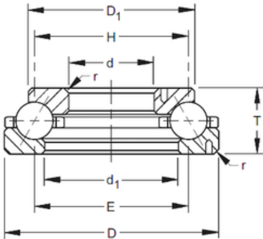
Bearing No. 245TVL716
